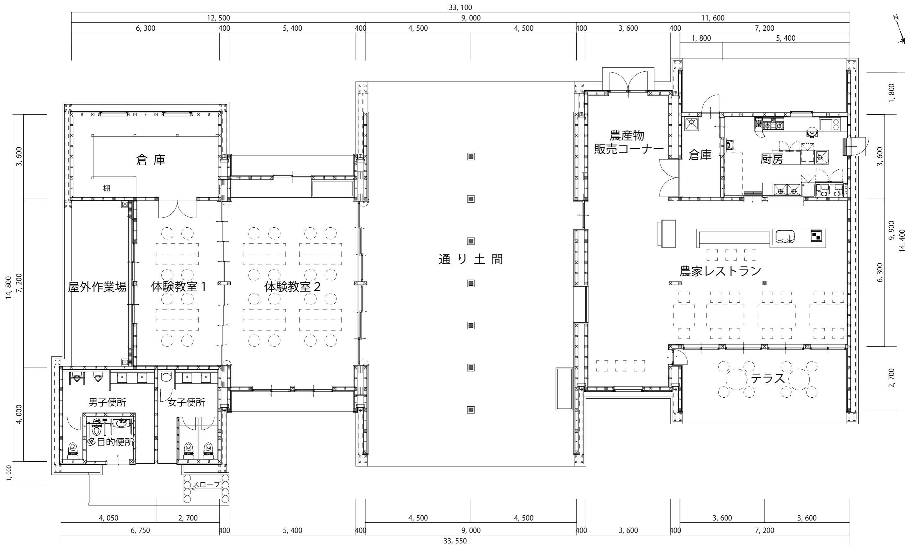
交流施設設計画図
